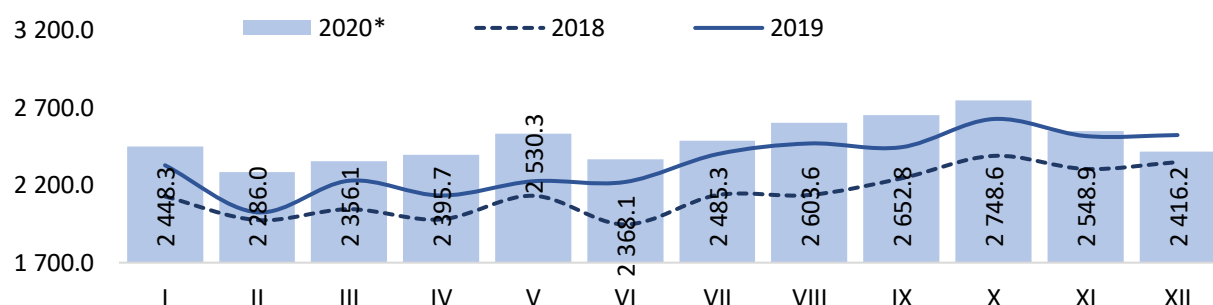
Зураг 16. Агаарын тээврээр тээсэн ачаа, тонн, сараар
