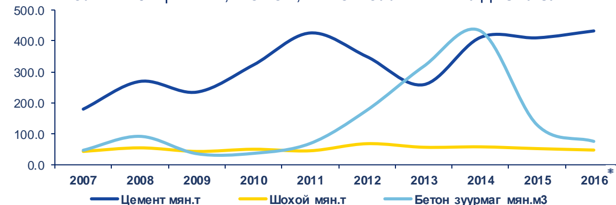
ЗУРАГ 15. ЦЕМЕНТ, ШОХОЙ, БЕТОН ЗУУРМАГ ҮЙЛДВЭРЛЭЛ
